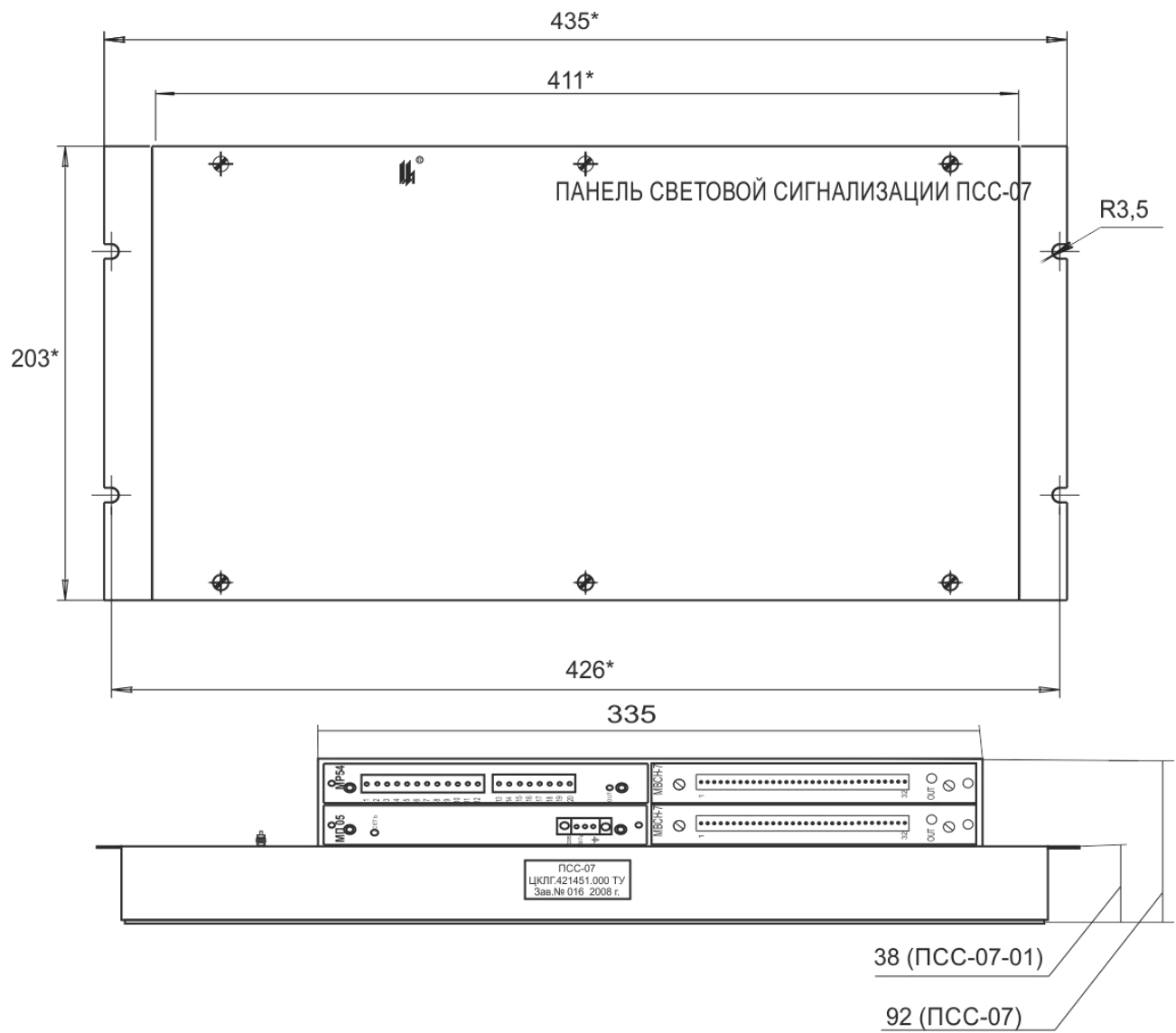
Рисунок Б.1 – Габаритные размеры ПСС-07
