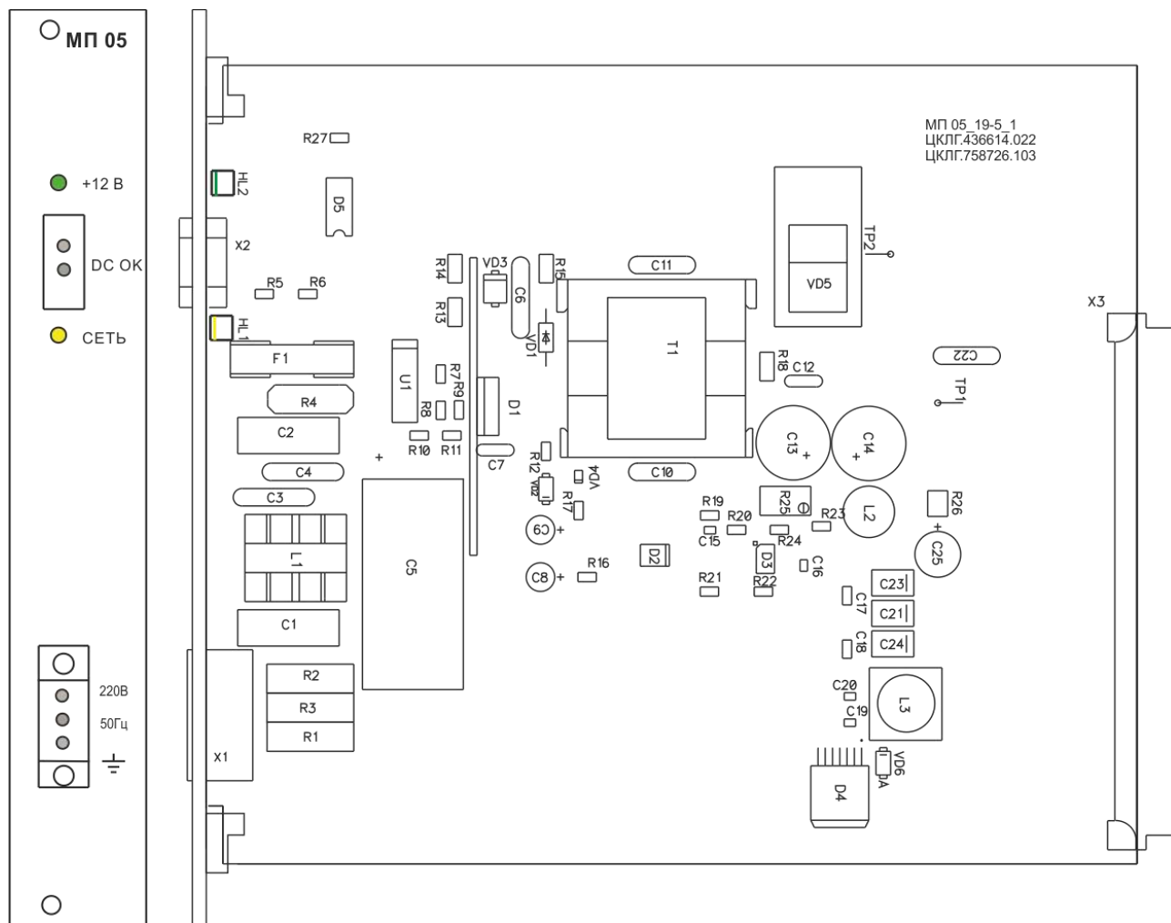
Рисунок 4.9 – Внешний вид печатной платы модуля питания МП-05
