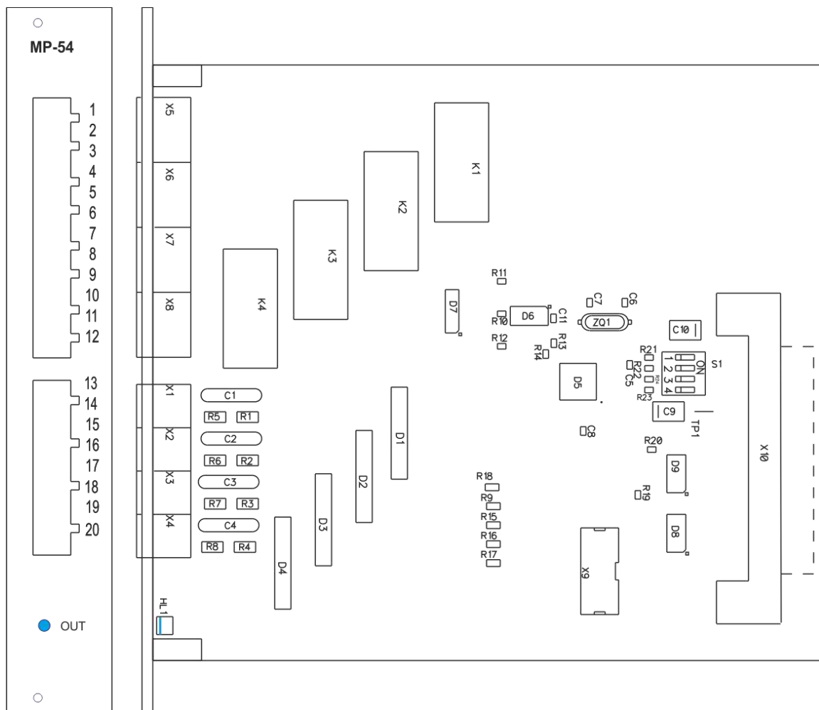
Рисунок 4.10 – Внешний вид печатной платы модуля реле MP-54
