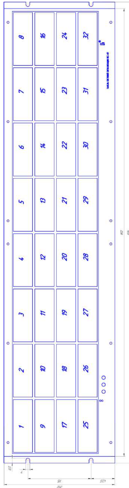
Рисунок Б.3 – Габаритные размеры ПСС-07-08
