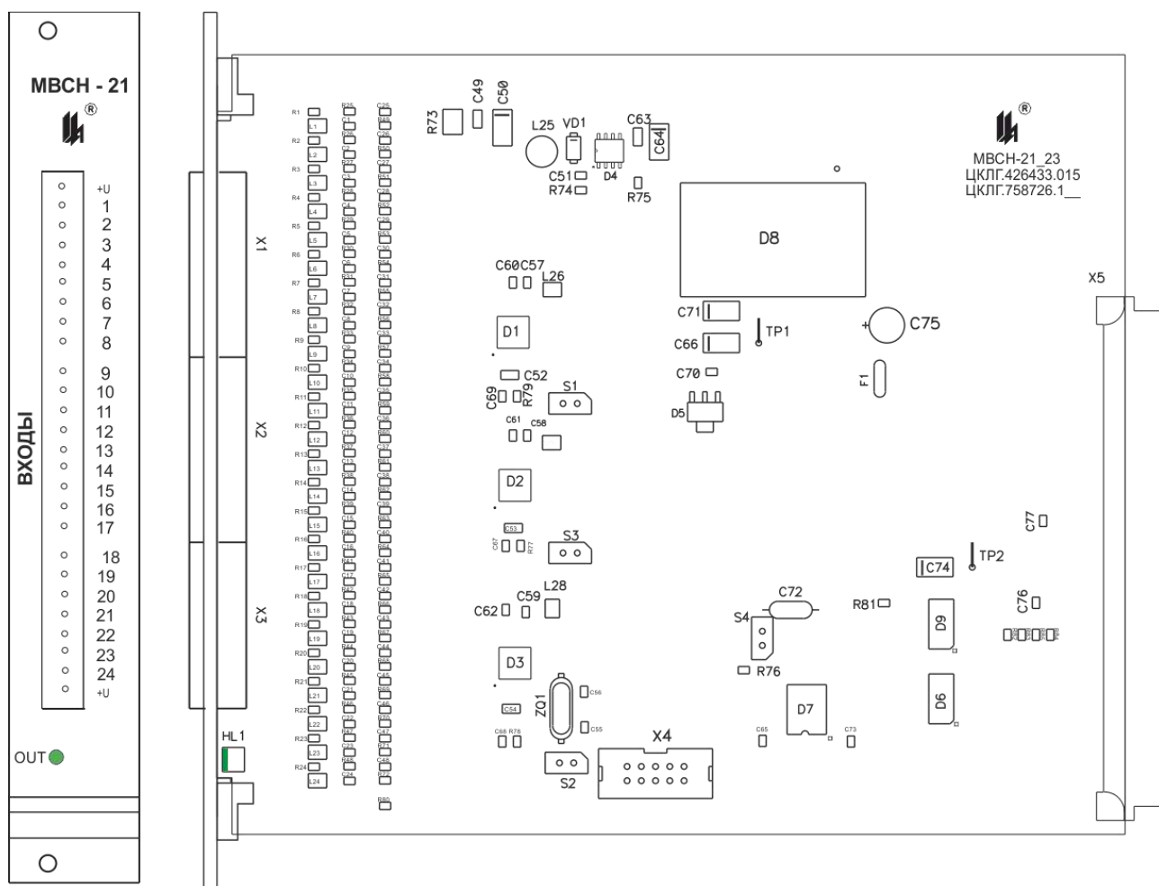
Рисунок 4.8 - Внешний вид платы модуля MBCH-21
