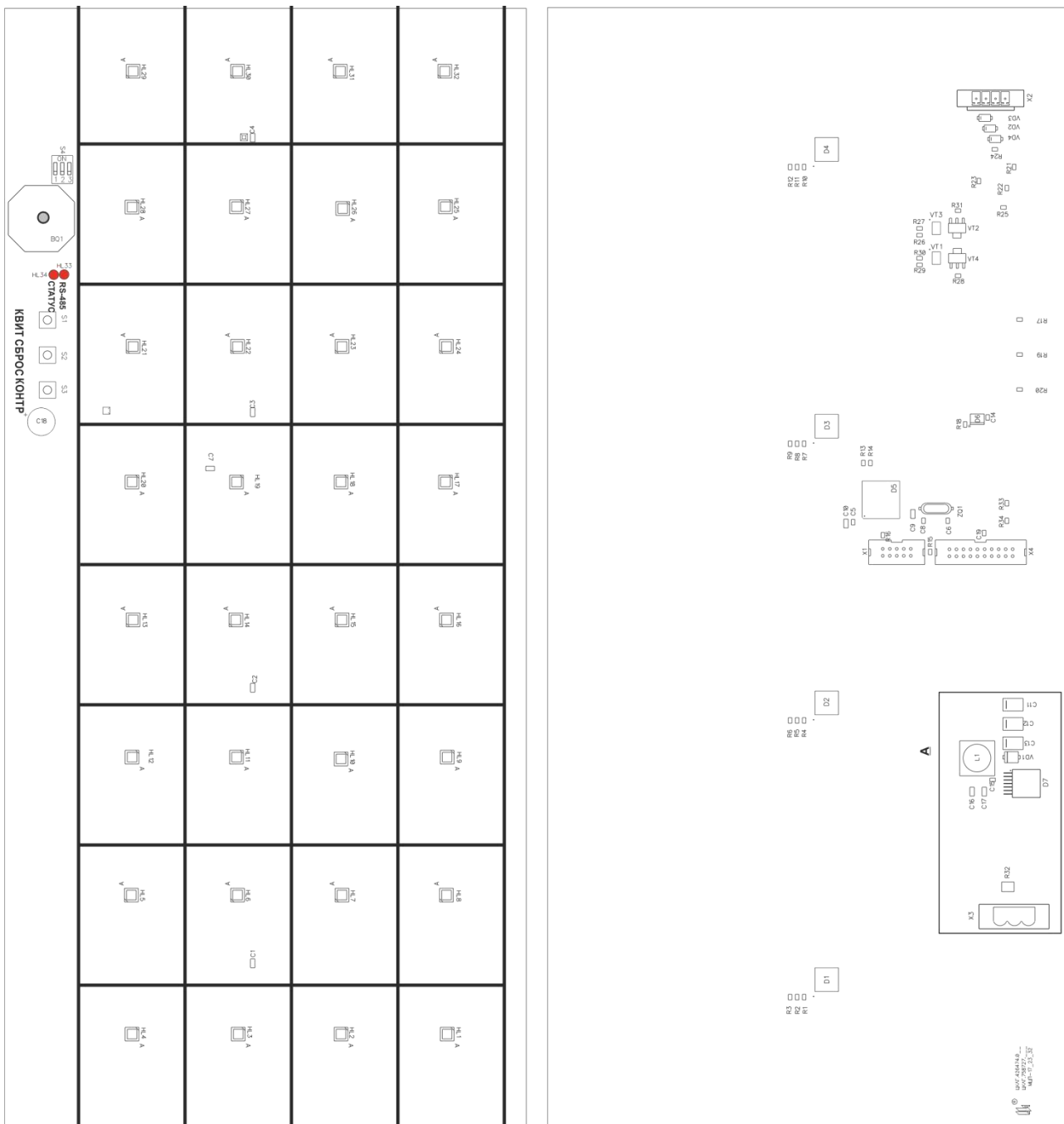
Рисунок 4.6 - Внешний вид печатной платы МЦП-17-16
