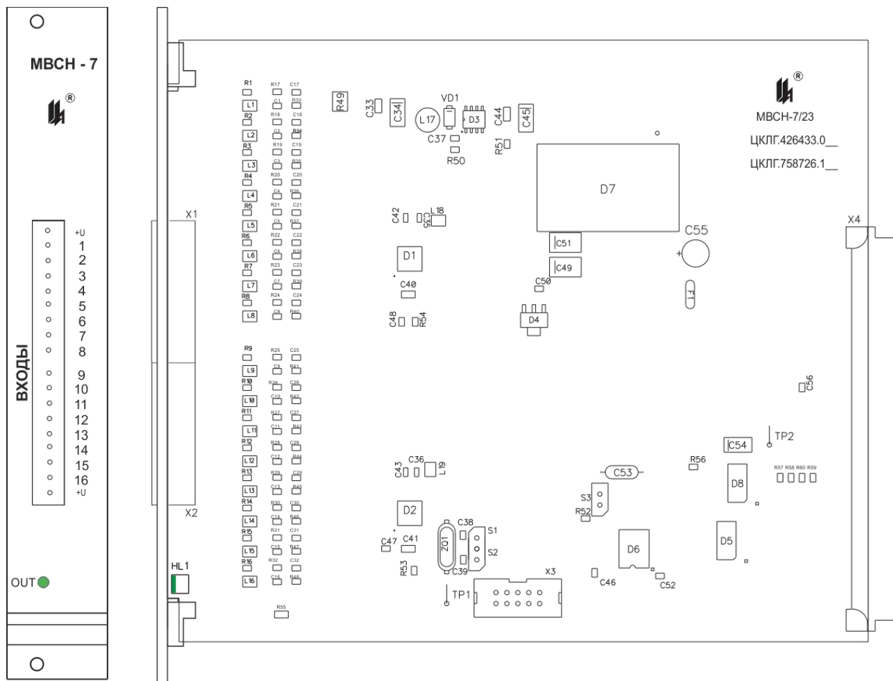
Рисунок 4.7 - Внешний вид платы модуля МВСН-7
