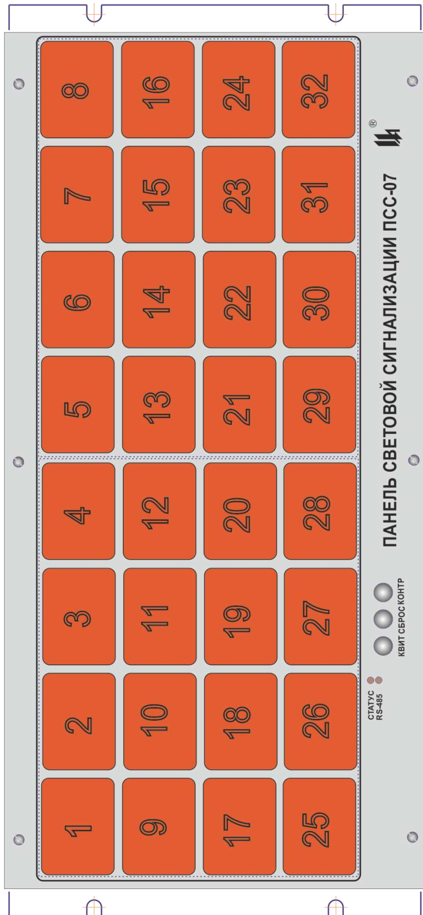
Рисунок 4.1 - Внешний вид ПСС-07 на 32 окна сигнализации 50 × 38 мм (в ПСС-07-04 и ПСС-07-05 светофильтр бесцветный)
